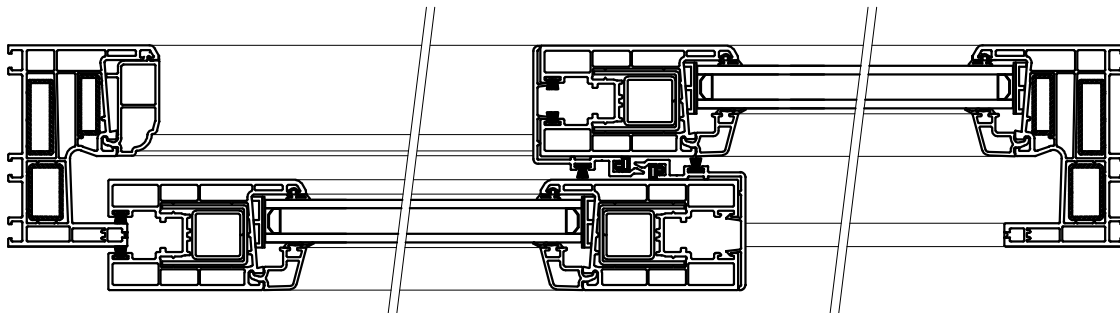
DETALLE 2
