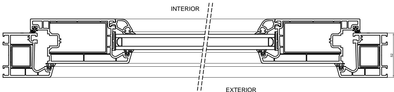
DETALLE 2
