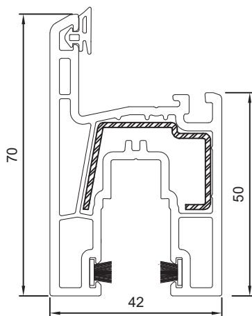
Hoja corredera 7461
