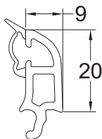
Junquillo para vidrio 20mm 7464
