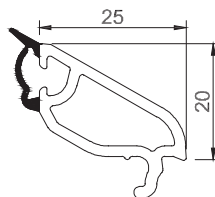
Junquillo para vidrio 4mm 7062
