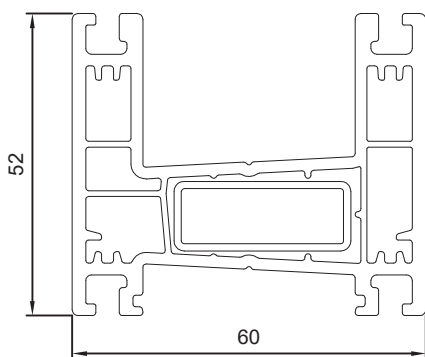
Marco corredera 2 hojas 7460
